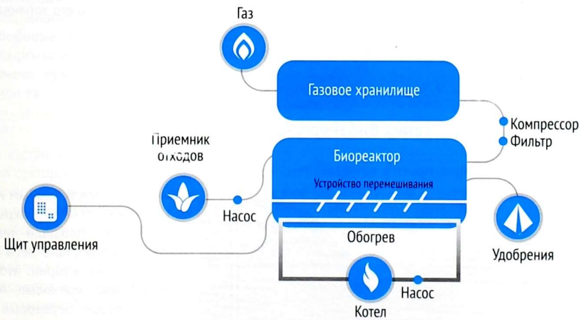
Рисунок 2.43. Схема устройства биогазовой установки
