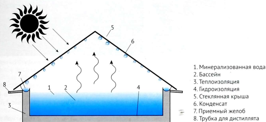
Рисунок 2.15. Солнечный дистиллятор-бассейн
