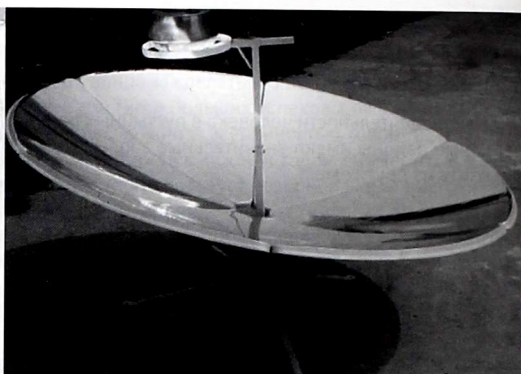
Рисунок 2.18. Солнечная печь из параболической антенны
