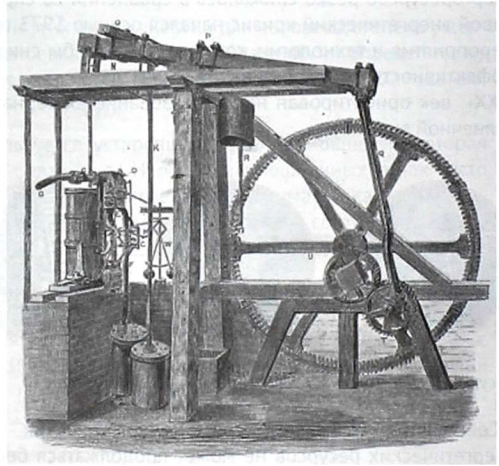
Рисунок 3.3. Паровая машина Джеймса Уатта
