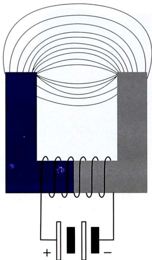
Рисунок 1.10. Образование электромагнитной энергии
