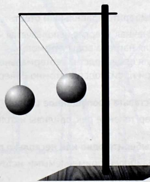
Рисунок 1.21. Нитяной маятник
