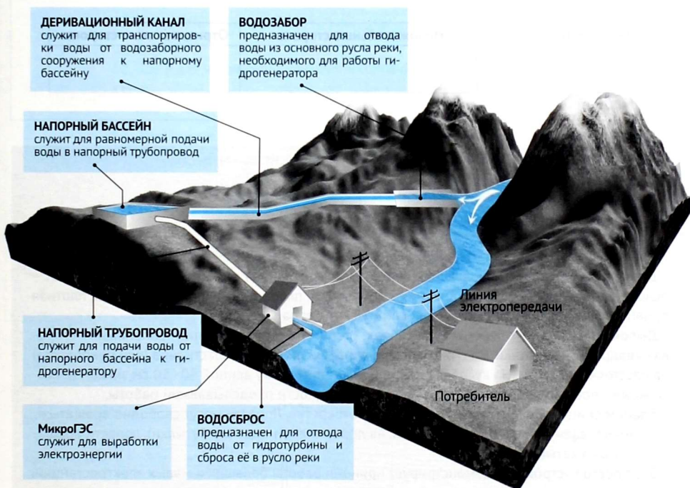
Рисунок 2.57. Принцип действия малой ГЭС 2
