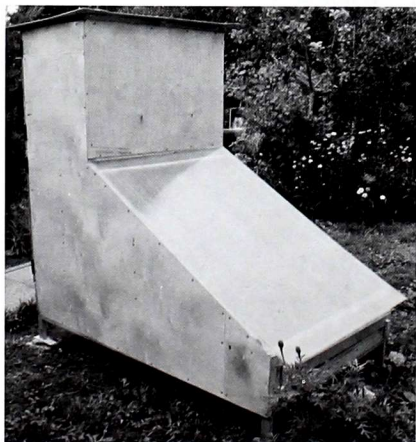
Рисунок 2.19. Солнечная сушилка
