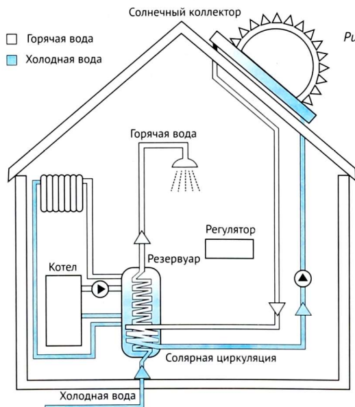
Рисунок 2.32. Система отопления с использованием солнечных коллекторов
