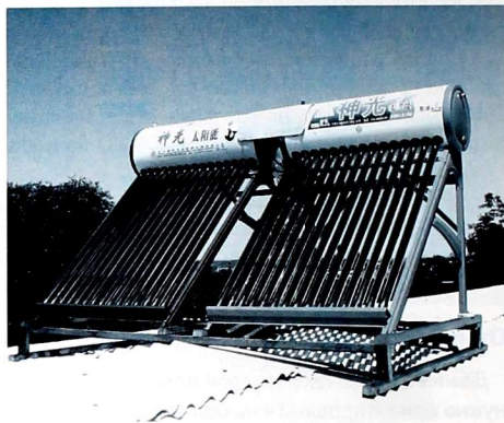
Рисунок 2.31. Солнечный коллектор на крыше дома
