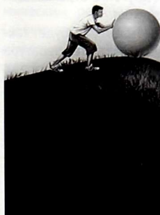
Рисунок 1.4. Камень, находящийся на краю обрыва, обладает потенциальной энергией 1 .
