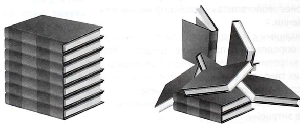
Рисунок 1.20. Иллюстрации второго закона термодинамики
