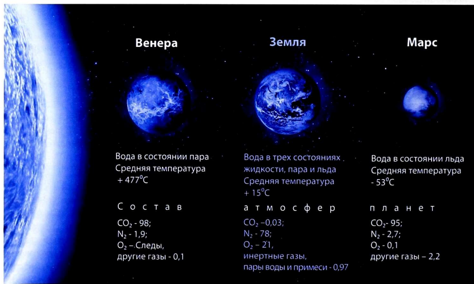
Рисунок 5.2. Основные компоненты атмосфер некоторых планет Солнечной системы 4
