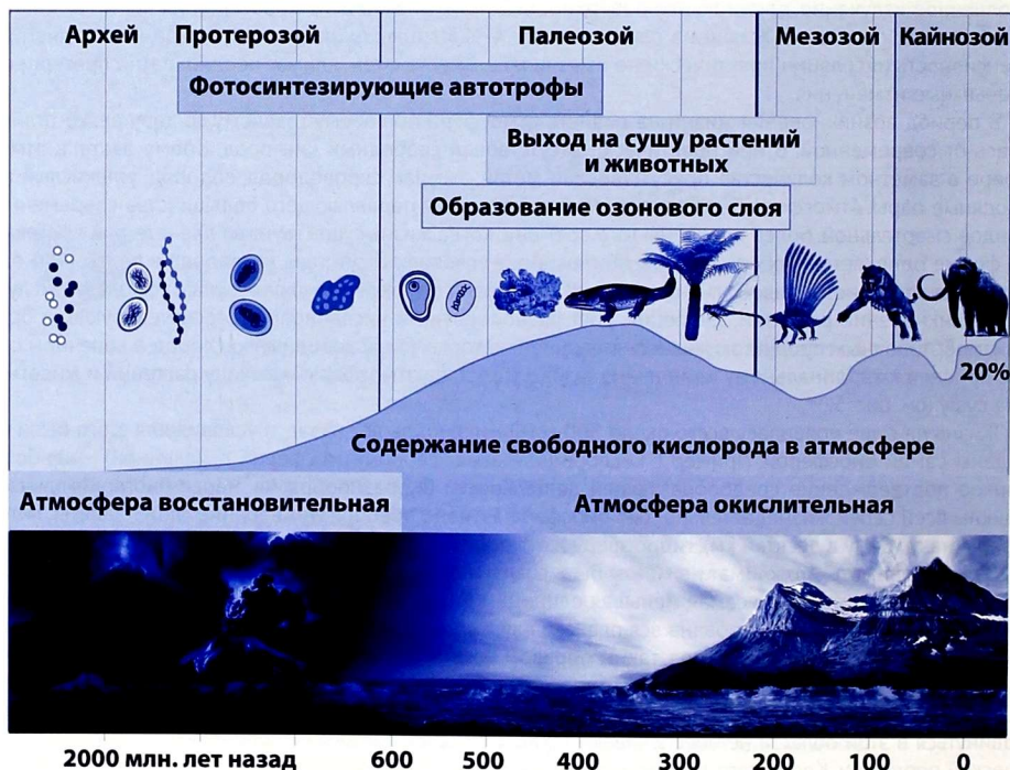
Рис. 5.3. Смена типов атмосфер и появления возможности выхода на сушу высших растений и животных как результат жизнедеятельности фотосинтезирующих автотрофов 2 .
