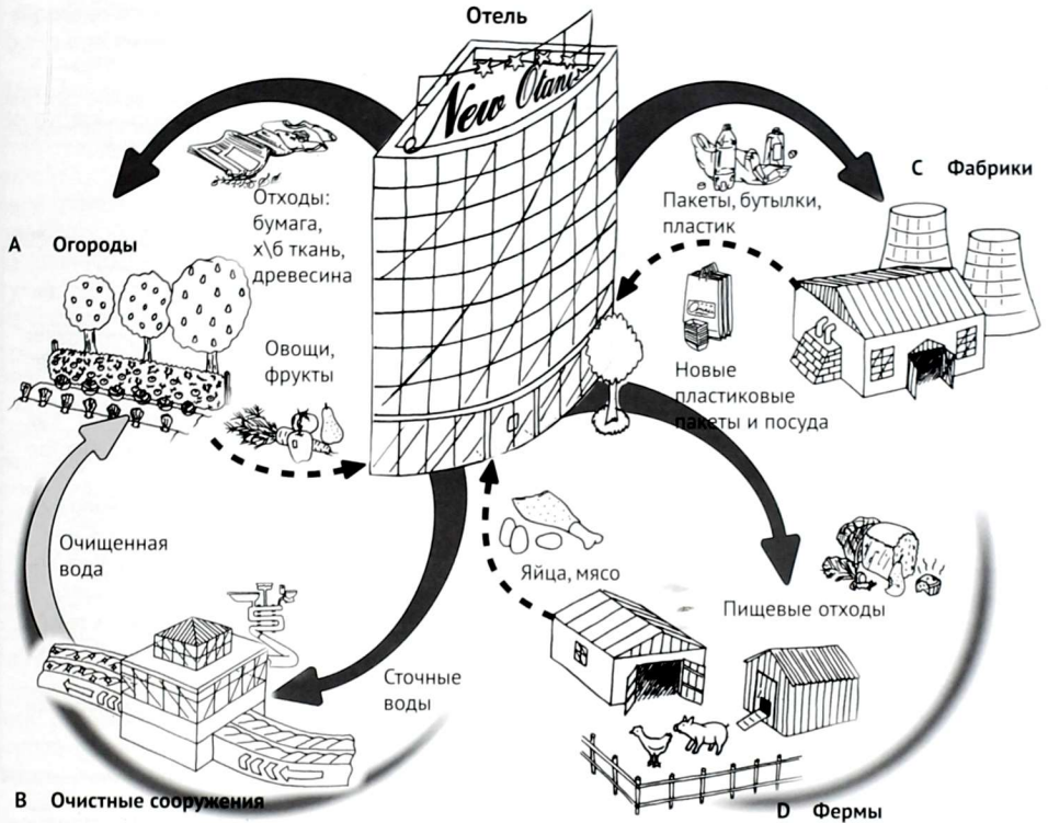
Рисунок 4.4. 1 Модель замкнутого экологического цикла
