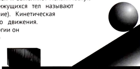
Рисунок 1.3. Пример использования кинетической энергии
