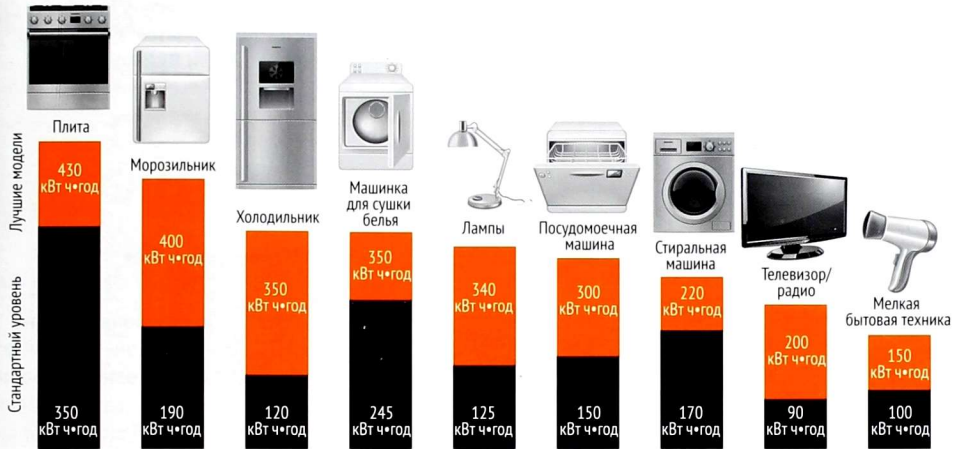
Рисунок 3.14. Годовые значения энергопотребления наиболее распространенных бытовых приборов для стандартных моделей, лучших по энергоэффективности
