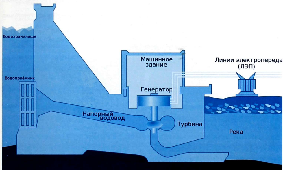
Рисунок 2.52. Устройство работы ГЭС
