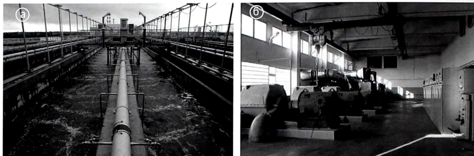
Рисунок 3.12. Очистка сточных вод: а – сооружение для очистки сточной воды с использованием микроорганизмов; б – устройство для подачи воздуха (воздуходувка)
