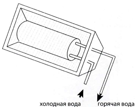
Рисунок 2.25. Солнечная бочка
